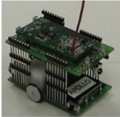
Resim 2.24: Açık kaynaklı minyatür sürü robotlar
